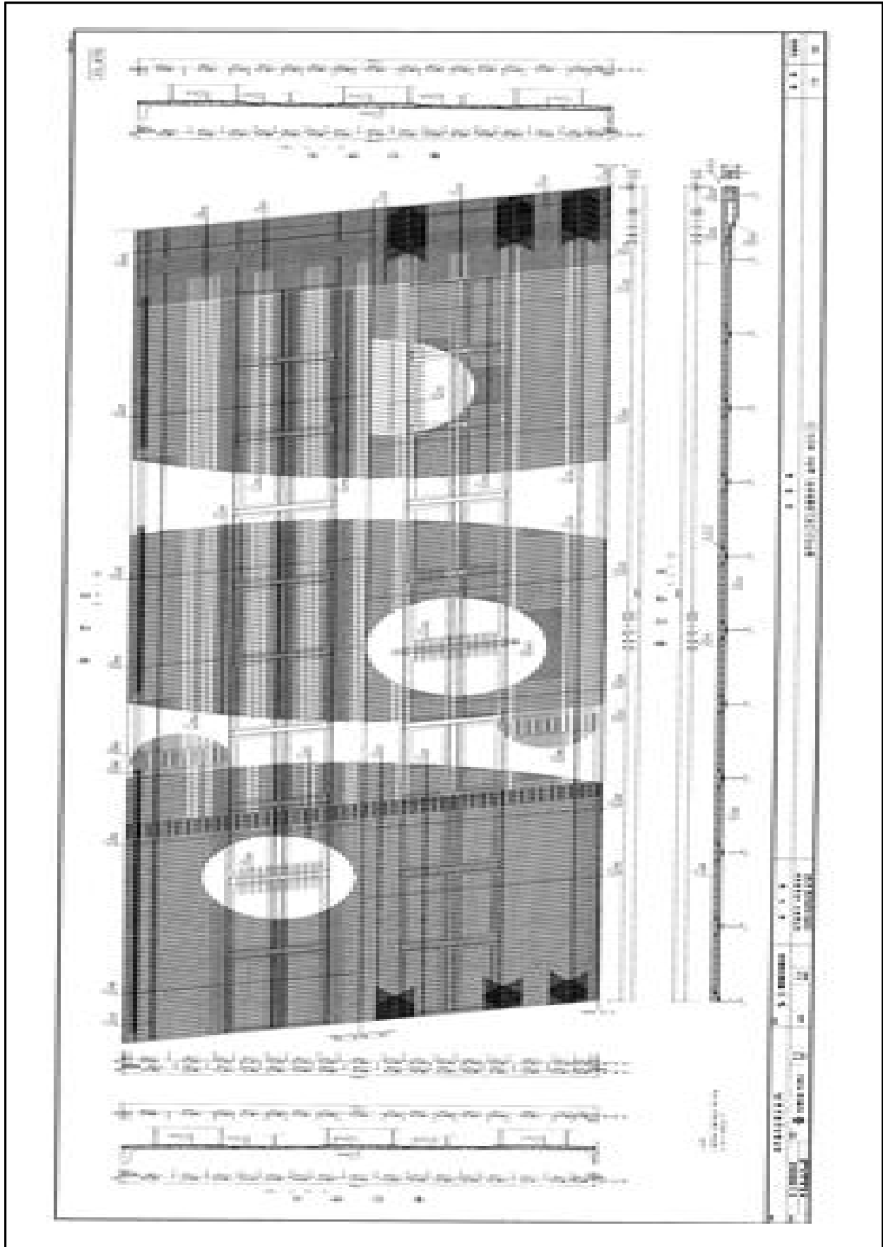
<그림 3.2.6> 배근도(슬래브)-계속
